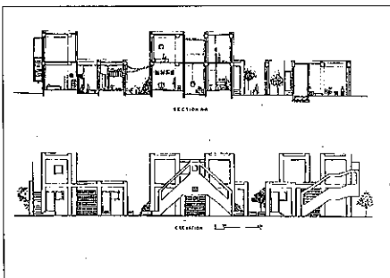
ユニット断面図
