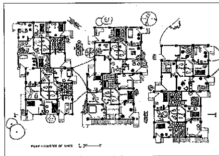
ユニット平面図
